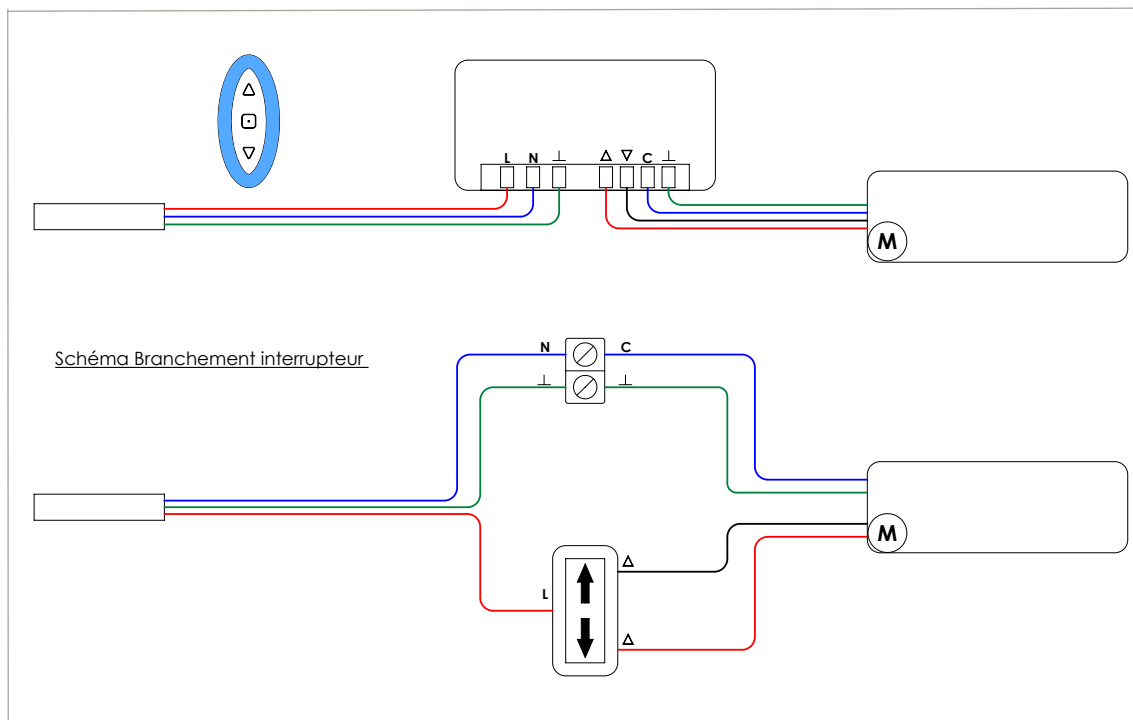
Schéma de branchement télécommande et interrupteur
