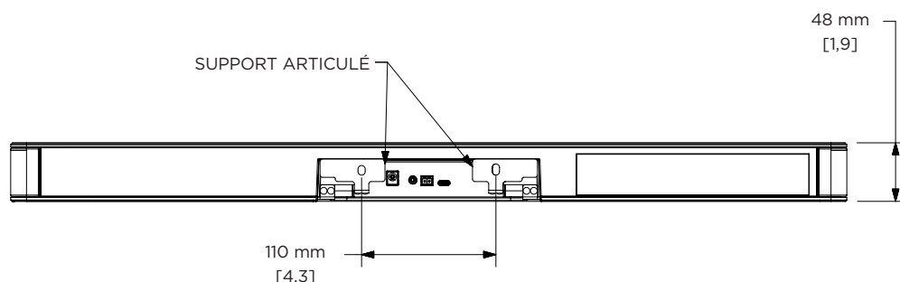
Vue arrière
