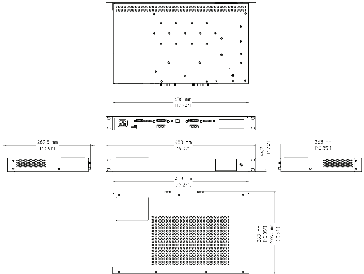
Fig. 3: Dimensions
