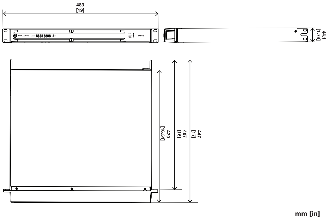
Fig. 4: Dimensions
