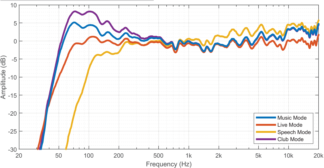
Fig. 2: Réponse en fréquence
