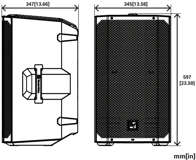
Fig. 1: Dimensions
